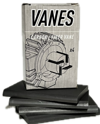
BR41710 - paletta in grafite mm. 70 x 43 x 6
